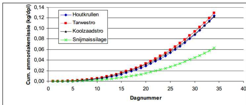
Figuur 6.2 Verloop ammoniakemissie bij de verschillende strooiselmaterialen op basis van modelpredictie
