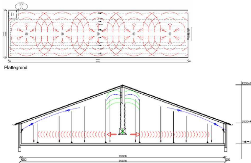
Figuur 6.1. Plattegrond en dwarsdoorsnede bij toepassen van stalsysteem V-6.3
